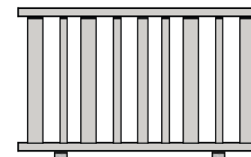
BERG : Lattes de 100mm Réf.612 alternées avec Barreaux rectangulaires 30x15mm Réf.1050 et Barreaux ovales 30x15mm Réf.311
