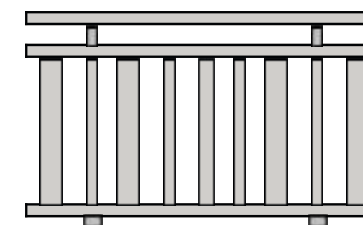
LOHR : Lattes de 100mm Réf.612 alternées avec Barreaux rectangulaires 30x15mm Réf.1050 et Barreaux ovales 30x15mm Réf.311
